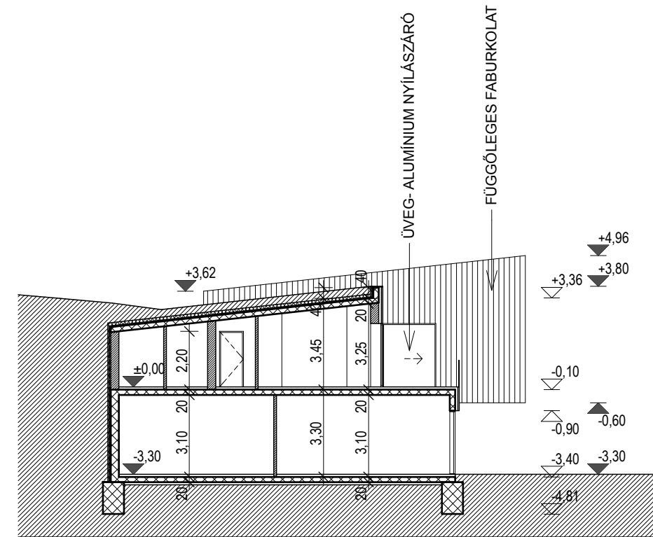
B-B METSZET
